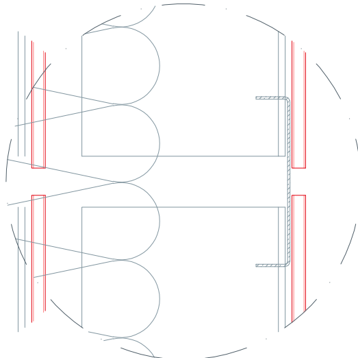
variante 2 fuga coperta (lamiera rivettata alla sottostruttura)
